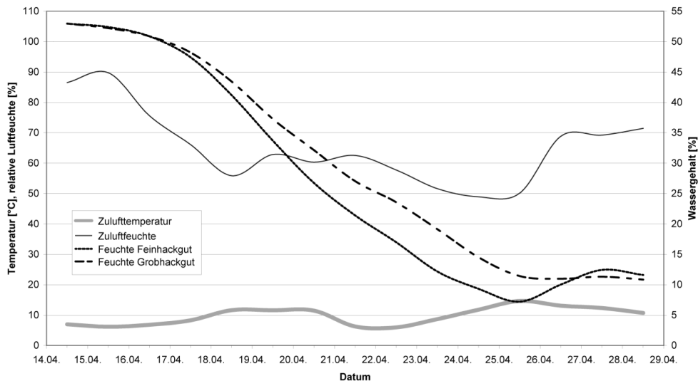
Trocknungsverlauf Holzhackschnitzel (Pappel)
